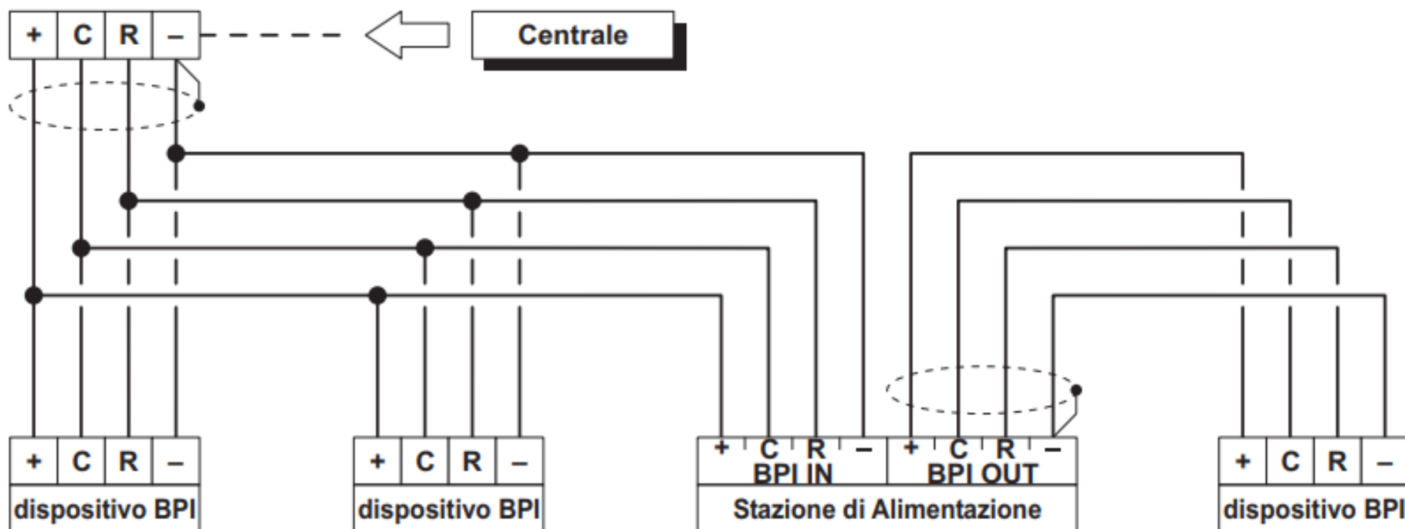
Figura 9 Collegamento di 4 Dispositivi BPI
